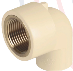
CODO HEMBRA DE CPVC CON INSERTO DE COBRE 1/2" X 90° 3/4" X 90° 3/4" X 1/2" X 90°
